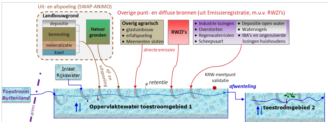
Figuur B1.1 Schematische weergave modelschematisering en modelinput nutriëntenbelasting oppervlaktewater.
