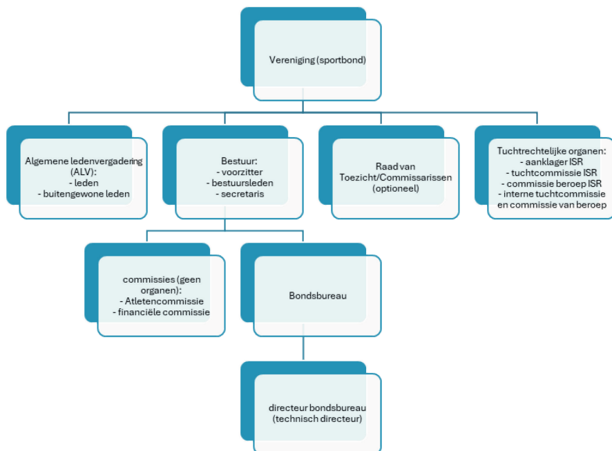
■ Figuur 2.2 Bondsstructuur
